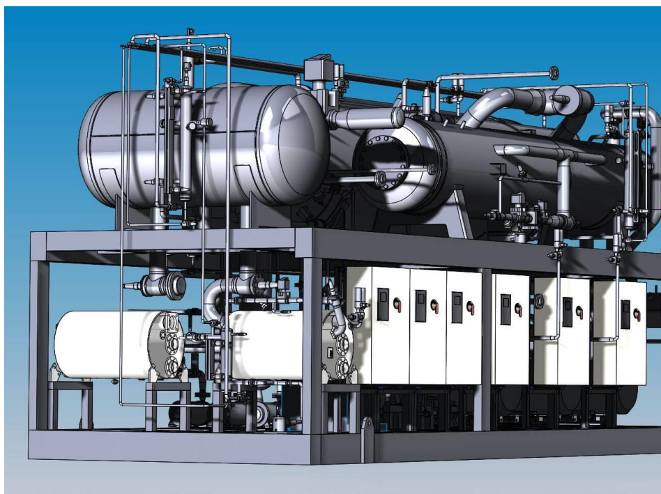
Рис.1.3 Аміачна компресорна
